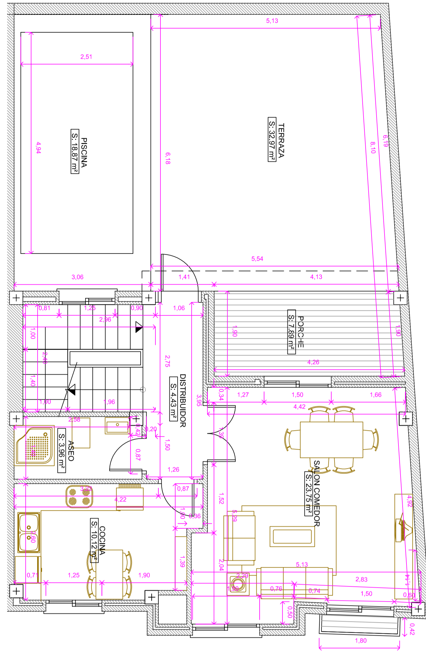
PLANTA PRIMERA
