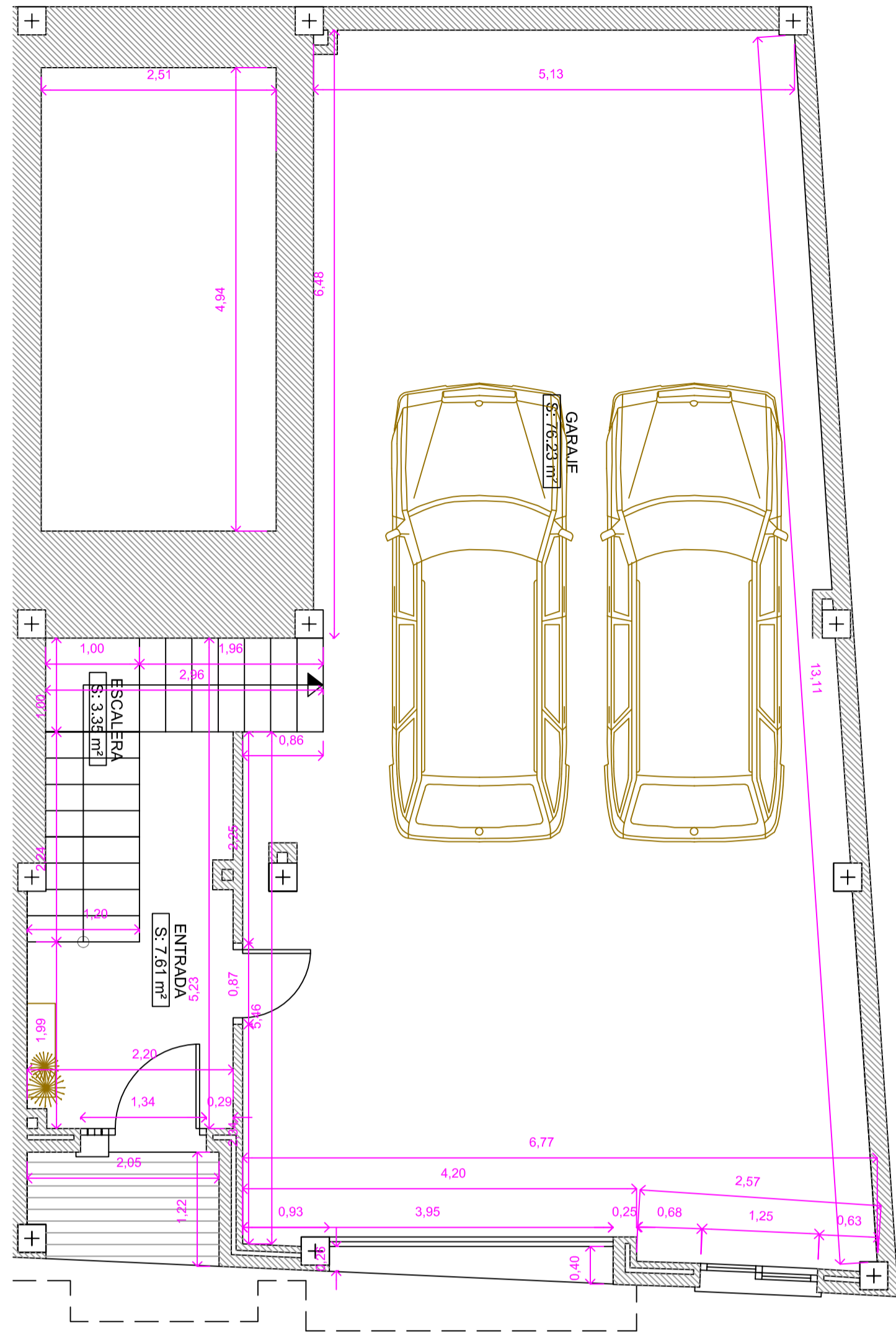
PLANTA BAJA
