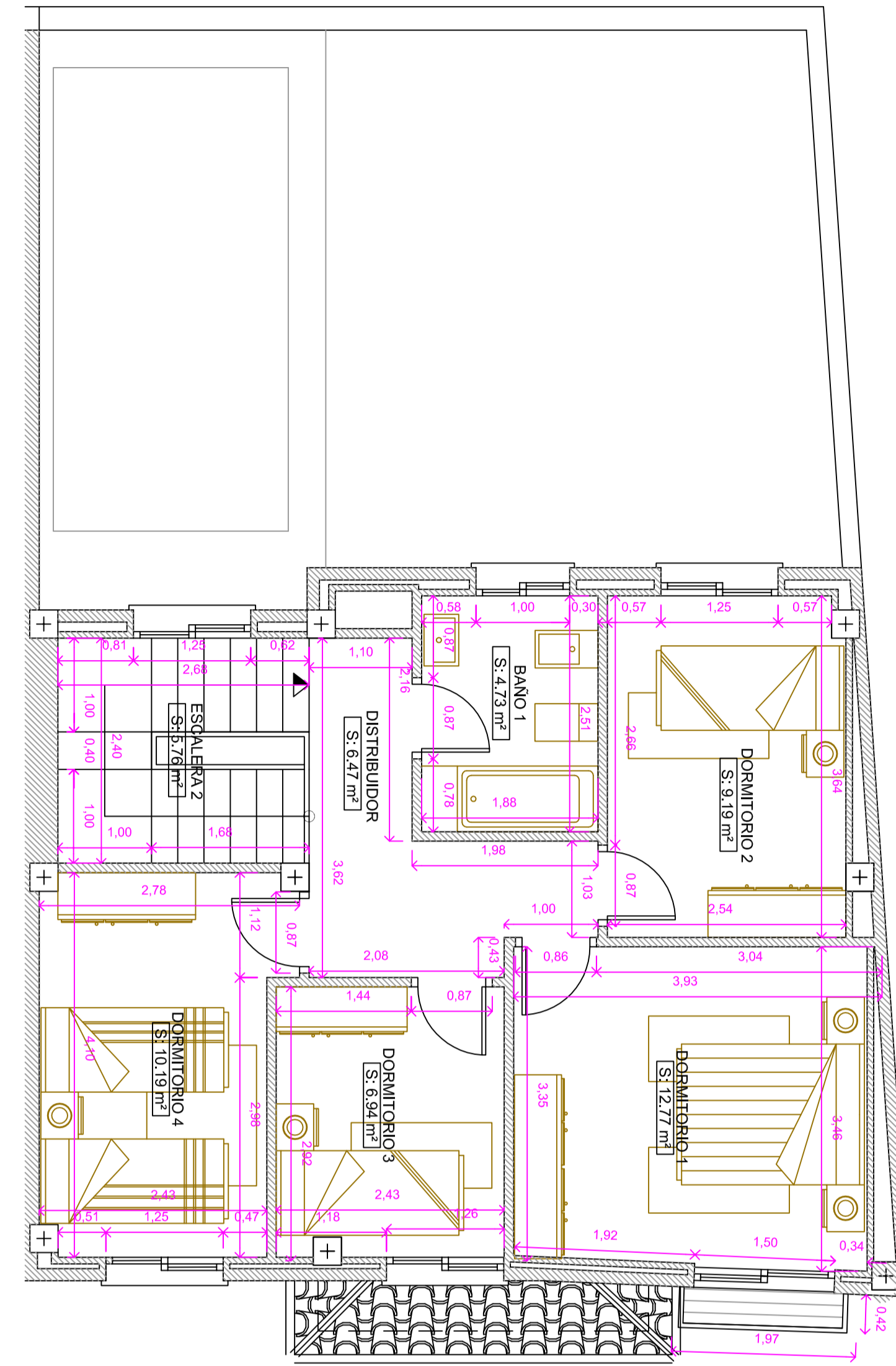
PLANTA SEGUNDA
